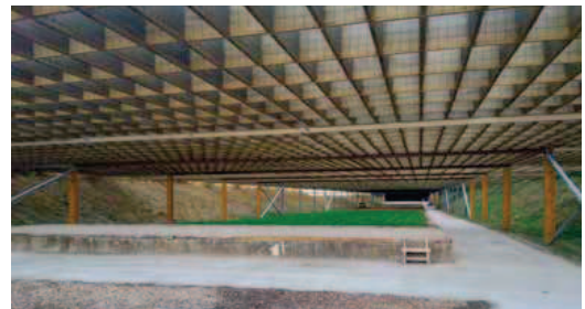
Den specielle konstruktion over skydebanen er opbygget af et stålskelet med plader af stenuld imellem.
